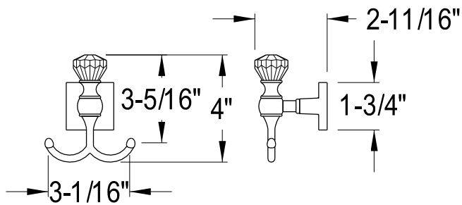
Robe Hook
